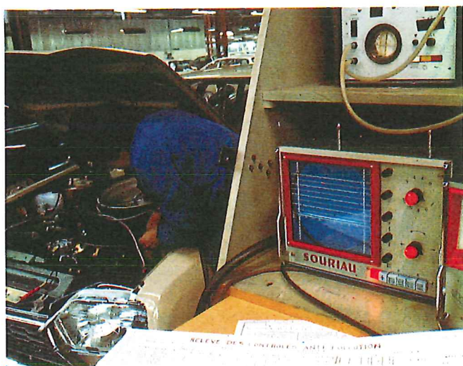
Contrôle de dépollution du moteur et réglages des taux d'oxyde de carbone et de gaz carbonique.
