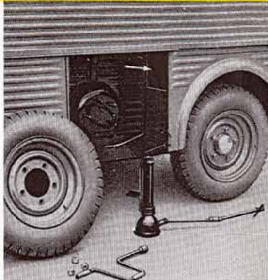
Lätt åtkomligt utrymme för reservhjul, dömkraft och verktygsutrustning.
