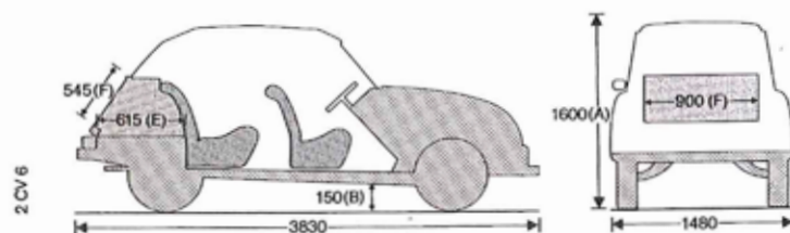
(A) Leeg (B) Vol (E) Vloerlengte (F) Breedte deuropening
